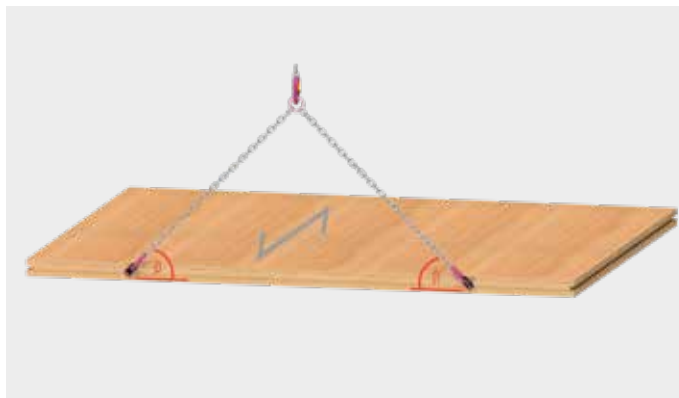
Parete o supporto BSH orizzontale, fibratura: verticale
