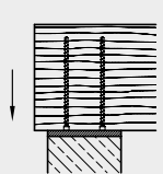
Rinforzo trazione trasversale dei collegamenti padiglione
