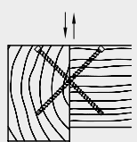
Rinforzo trazione trasversale su intagli
