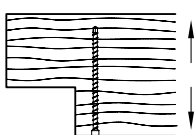
Rinforzo trazione trasversale su intagli
