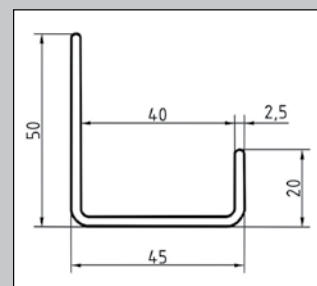
Disegno del profilo inferiore
