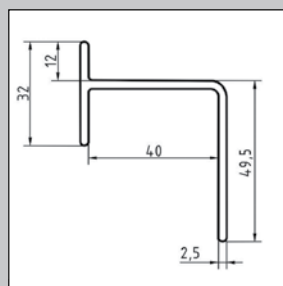
Disegno del profilo superiore
