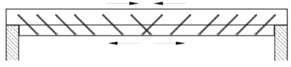
Rinforzo trazione trasversale dei collegamenti padiglione
