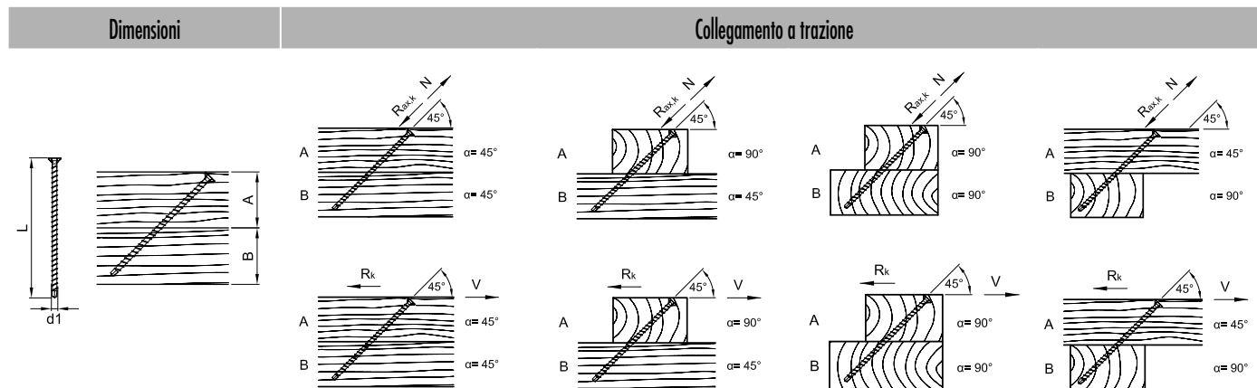
Valore caratteristico della portata della connessione R_{ax,k} e/o R_k secondo ETA-11/0024
