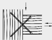
Rinforzo trazione trasversale su fresatura passante
