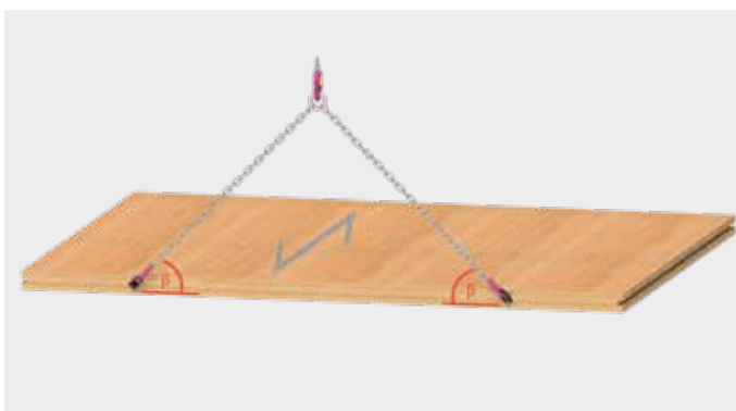
Parete o supporto BSH orizzontale, fibratura: verticale
