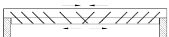
Zdwojenie belek
